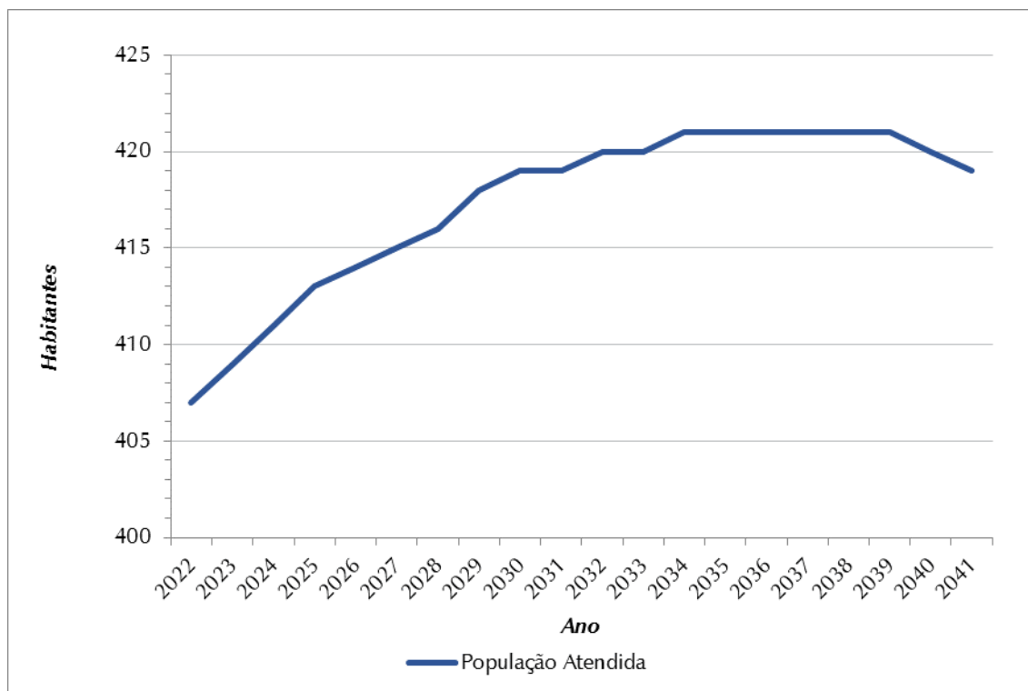
Figura 7.3 – Evolução da População Atendida (hab.) – SAA São Sebastião
