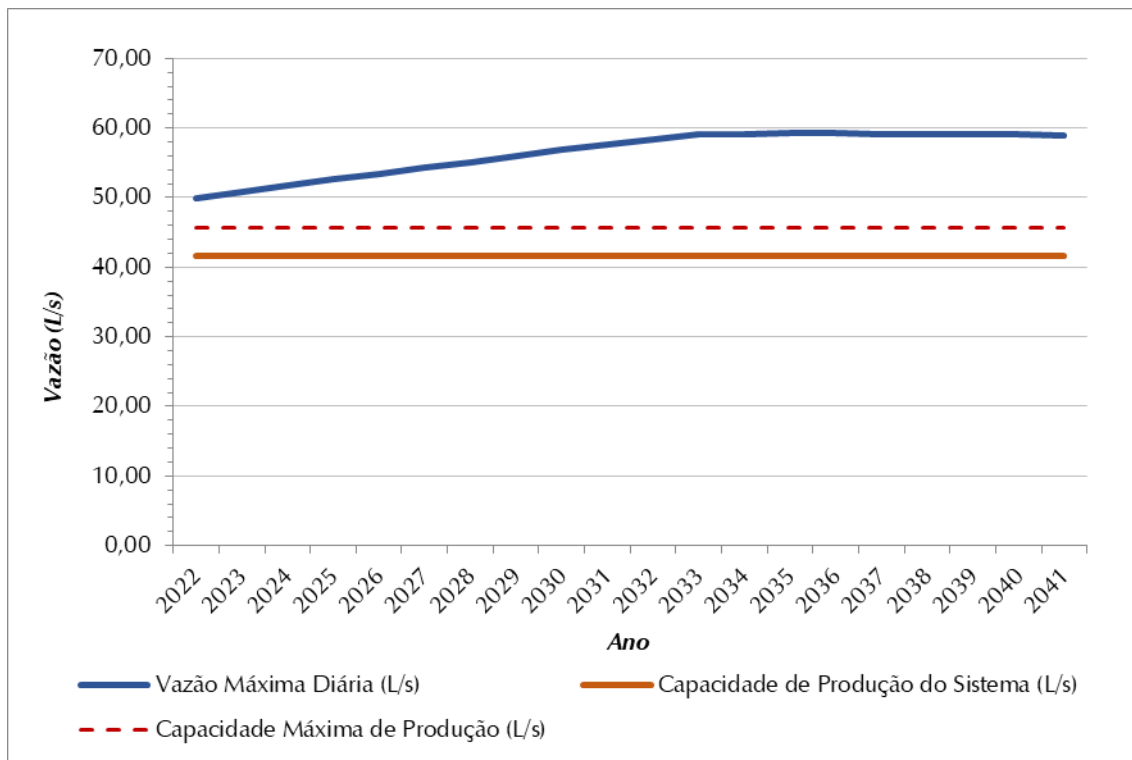
Figura 8.1 – Demandas Máximas Diárias (L/s) X Vazão Captada (L/s) – SAA Sede Total
