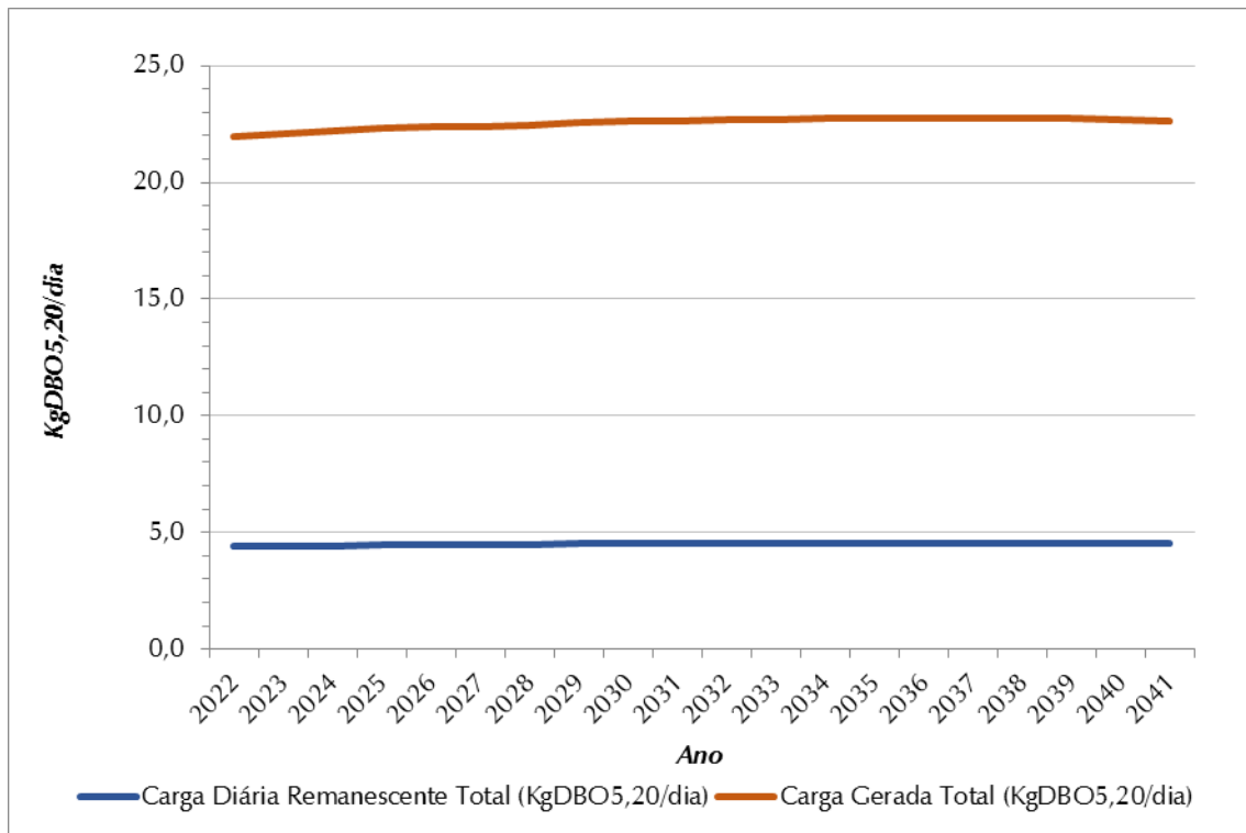
Figura 8.8 - Evolução de Cargas Orgânicas (Kg DBO 5,20 /Dia) – SES São Sebastião
