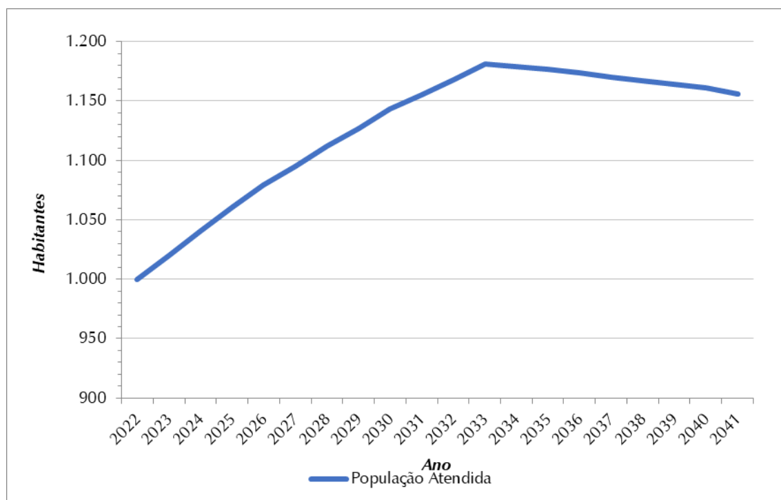
Figura 7.8 - Evolução da População Atendida (hab.) – SES Espigão
