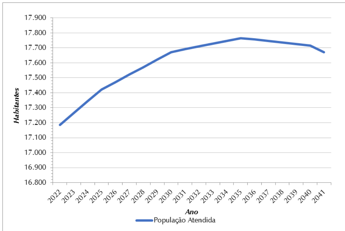
Figura 7.6 - Evolução da População Atendida (hab.) – SES Sede
