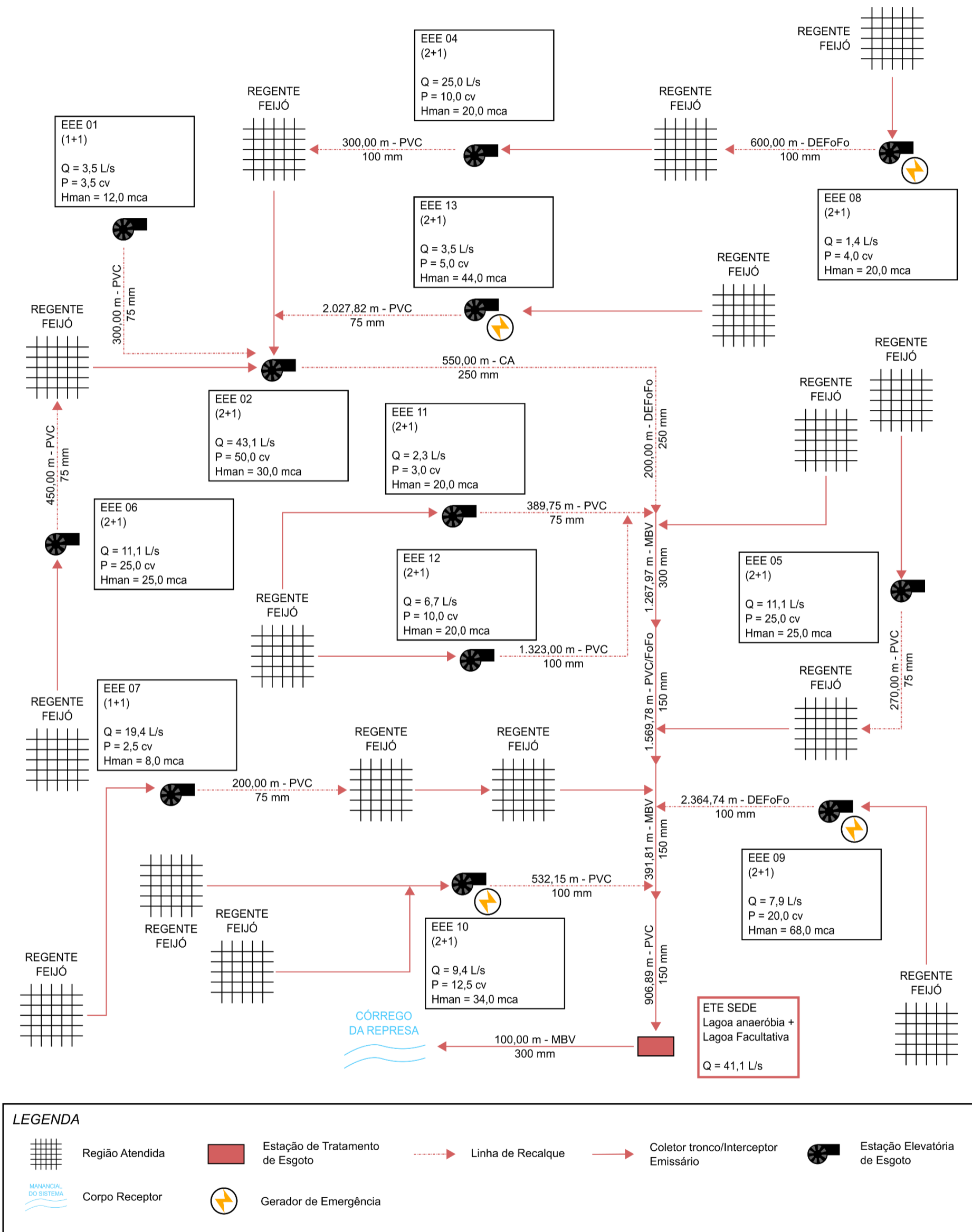
Figura 4.3 – Croqui do Sistema de Esgotamento Sanitário da Sede Fonte: SABESP, 2021.
