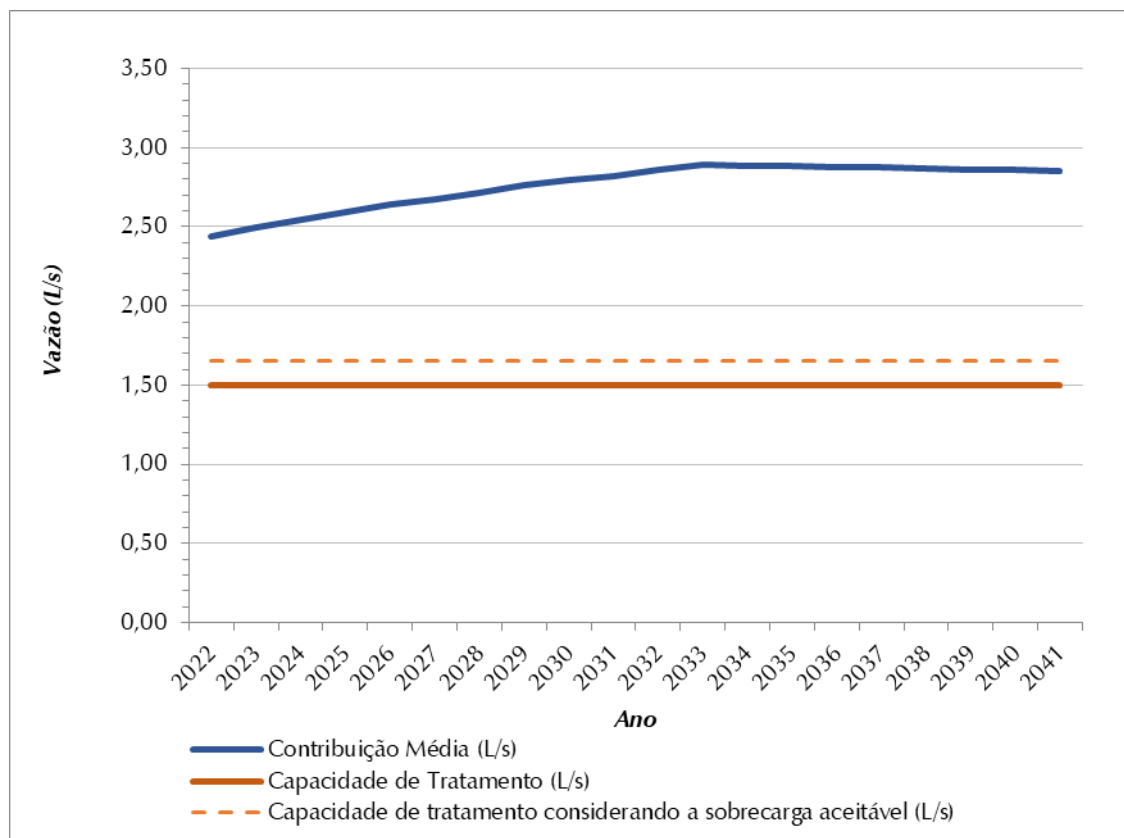
Figura 8.9 – Contribuição Média Total (L/s) x Capacidade de Tratamento de Esgoto (L/s) – SES Espigão
