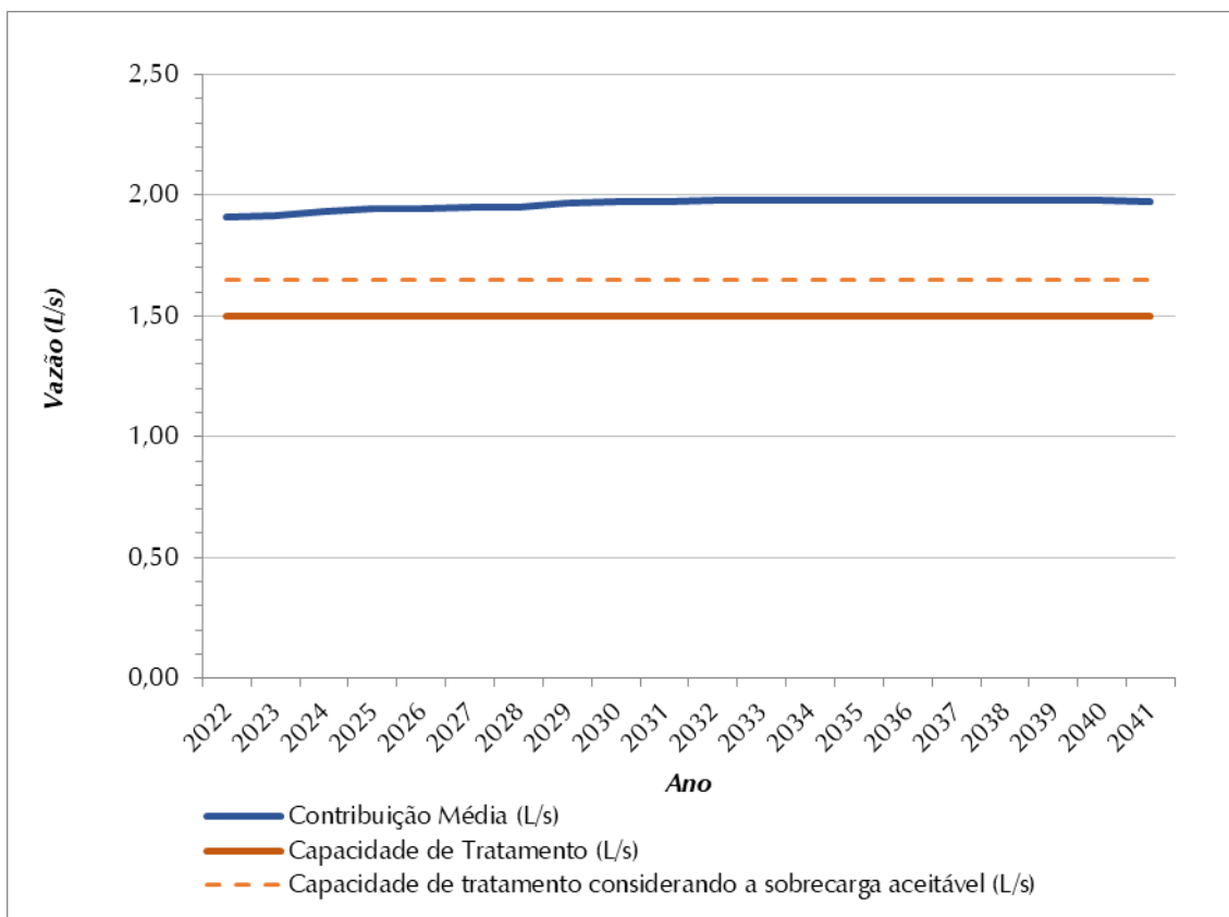
Figura 8.7 – Contribuição Média Total (L/s) x Capacidade de Tratamento de Esgoto (L/s) – SES São Sebastião
