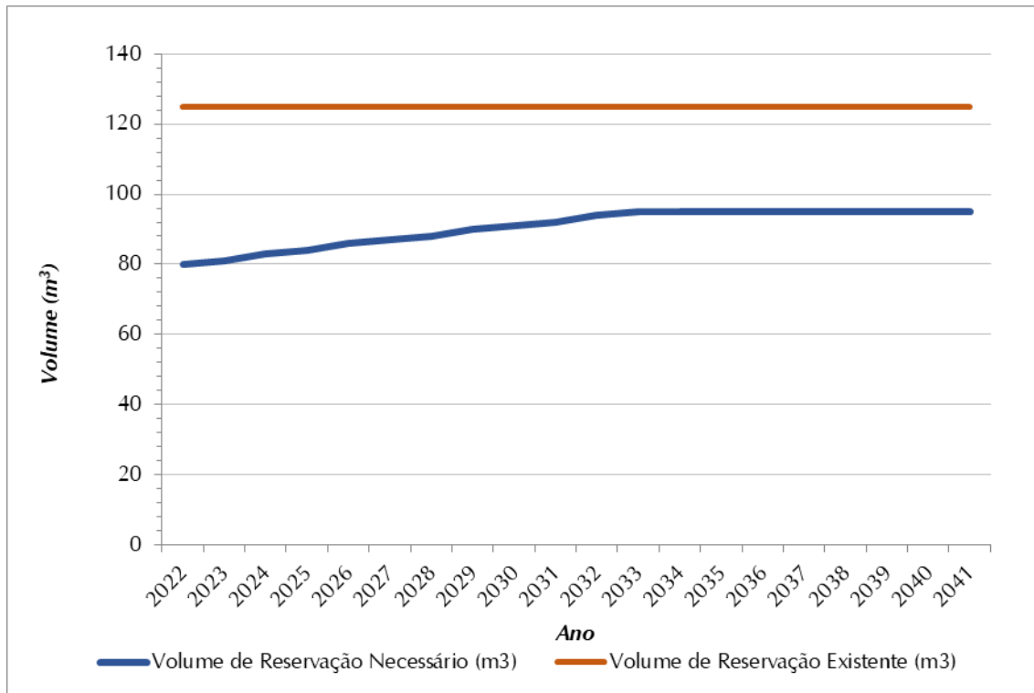
Figura 8.4 - Volume de Reservação Necessário (m³) x Volume de Reservação Atual (m³) SAA Espigão
