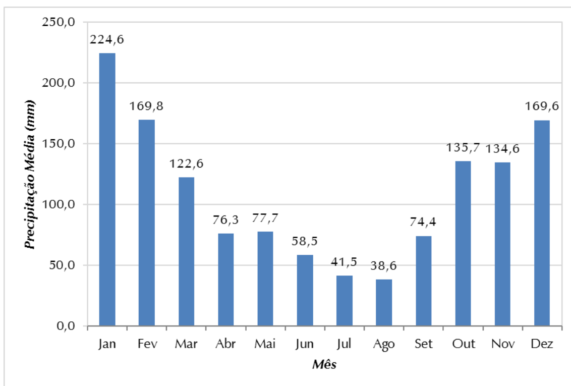
Figura 3.2 - Precipitação Média Mensal no Período de 1950 a 2021, Estação D8-047
