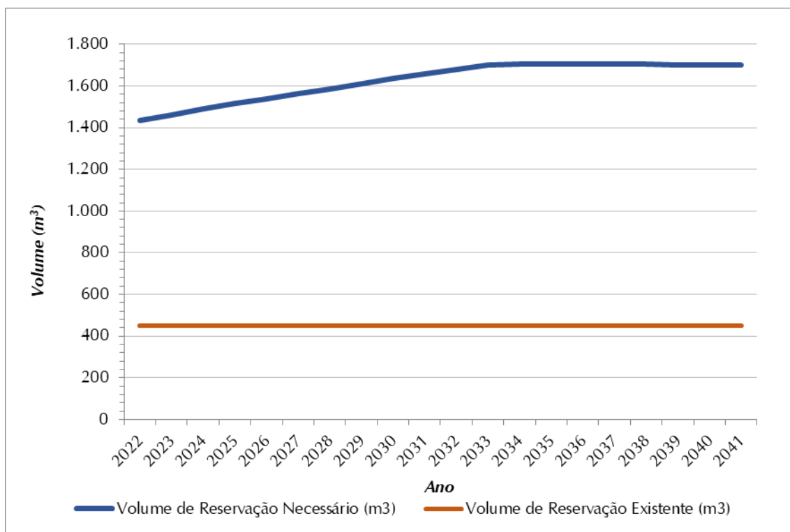
Figura 8.2 - Volume de Reservação Necessário (m³) x Volume de Reservação Atual (m³) – SAA Sede Total
