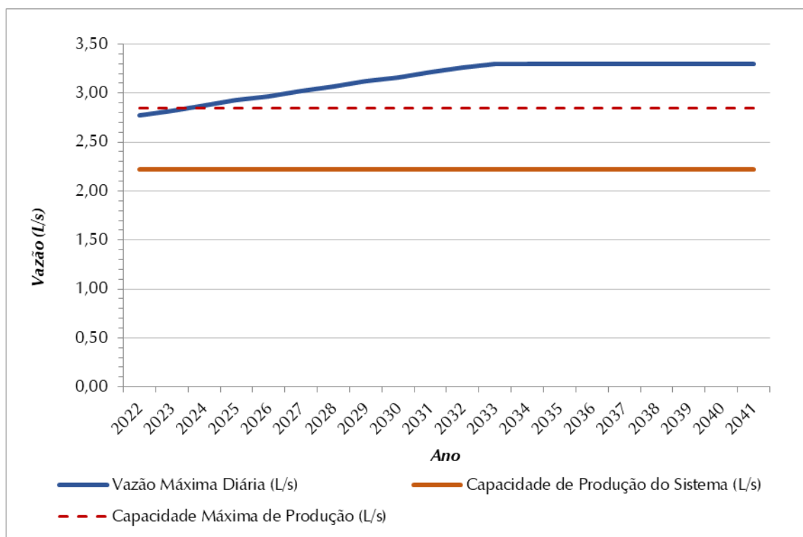
Figura 8.3 – Demandas Máximas Diárias (L/s) X Vazão Captada (L/s) – SAA Espigão
