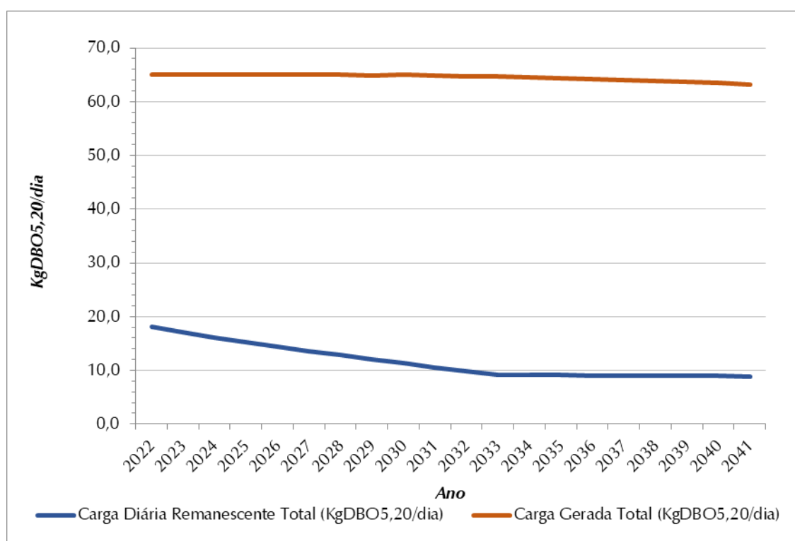
Figura 8.10 - Evolução de Cargas Orgânicas (Kg DBO 5,20 /Dia) – SES Espigão
