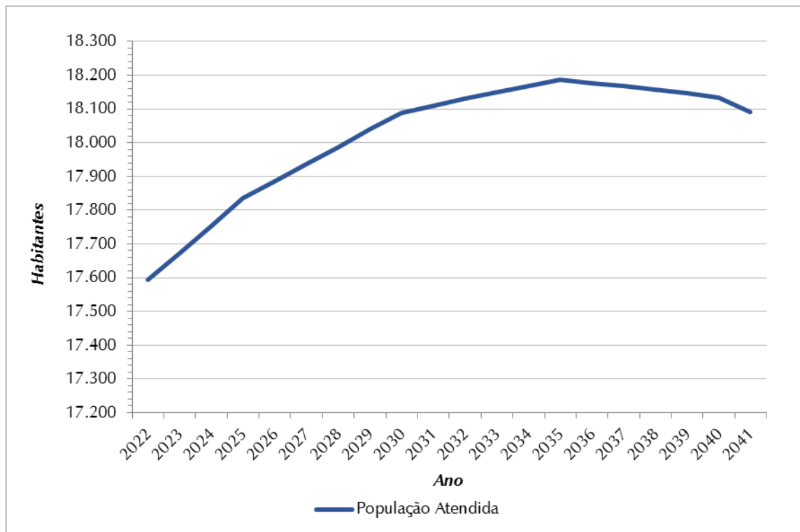
Figura 7.4 – Evolução da População Atendida (hab.) – SAA Sede Total
